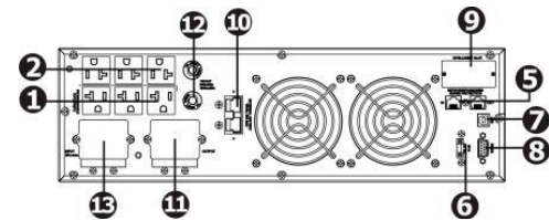
3KVA(機架式)
