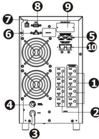
2KVA(直立式)
