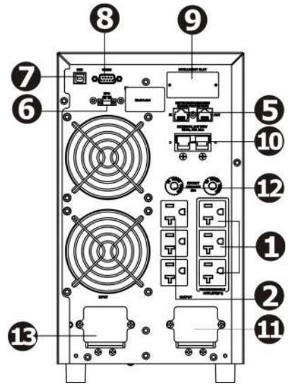
3KVA(直立式)
