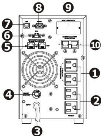
1KVA/1.5KVA(直立式)
