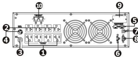
2KVA(機架式)
