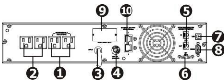
1KVA/1.5KVA(機架式)
